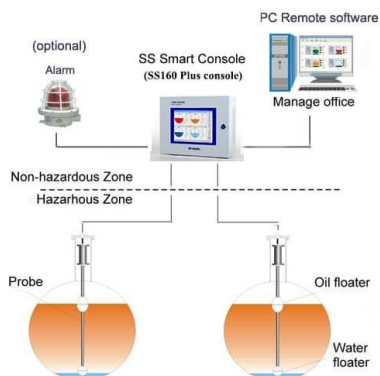
Système de jaugeage de cuves
